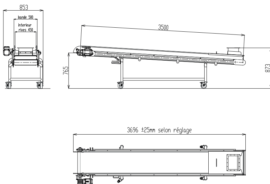
Plans du modèle SD-H 450-3500
