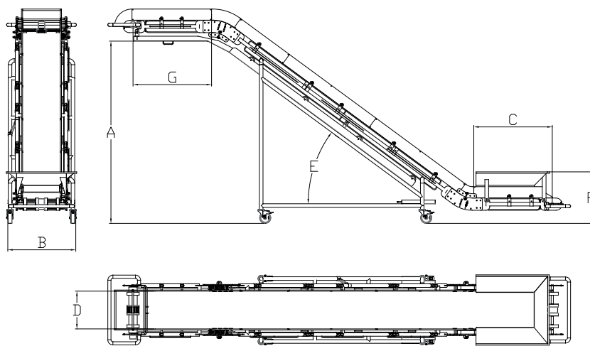
Plans du modèle DCDC-H
