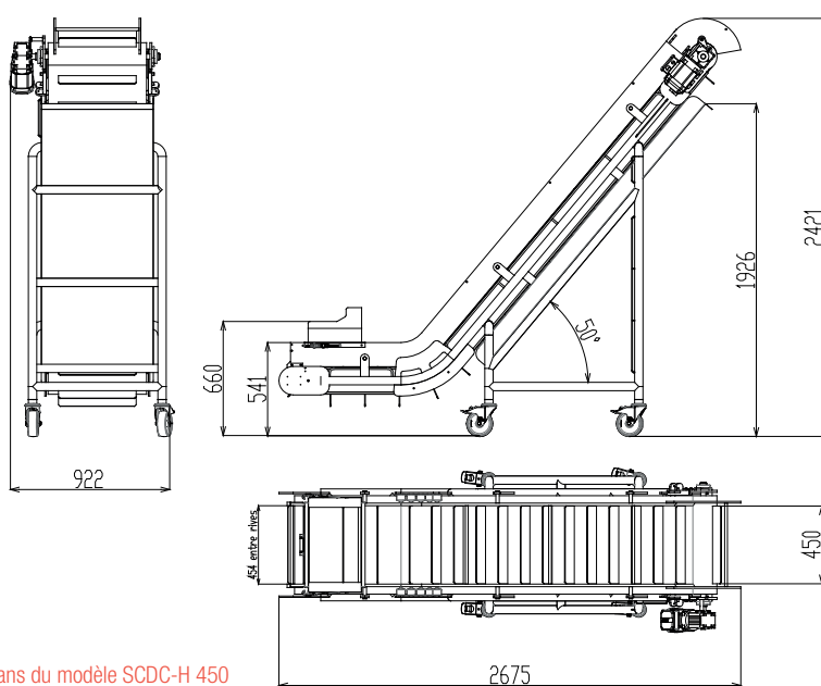
Plans du modèle SCDC-H 450
