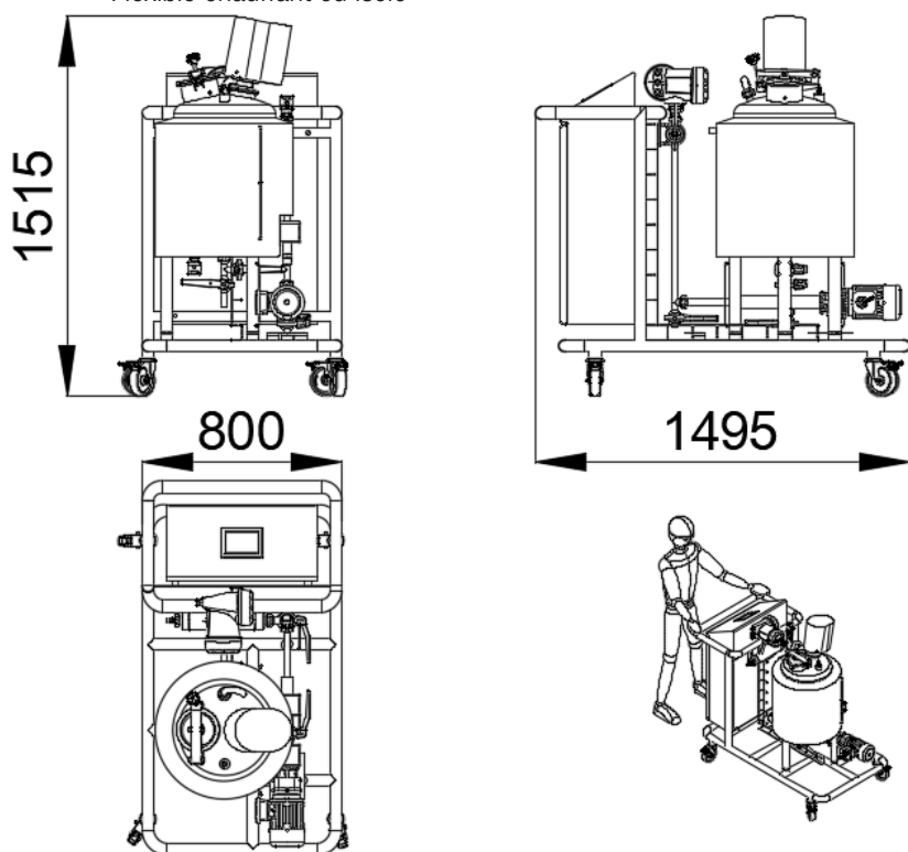
Plan du modèle SKDX100H
